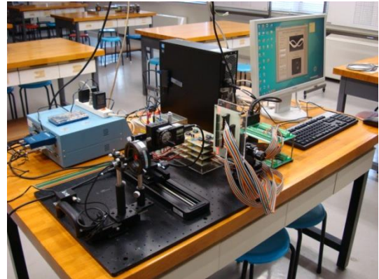
シングルヘリカル模擬CT装置の外観
