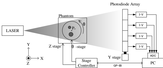
模擬CT装置の構成
